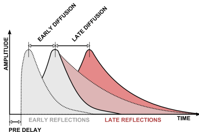
Сигнал реверберации
