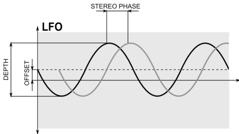
Сдвиг фаз между стерео каналами посредством LFO
